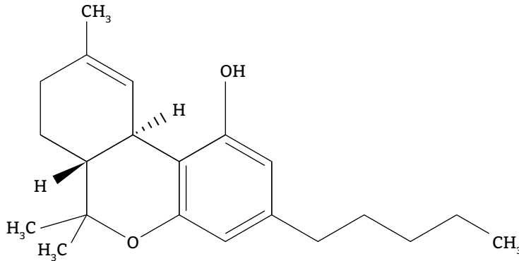
Figura N° 5. Estructura química de Δ9-tetrahidrocannabinol (THC. Fitocannabinoide)
